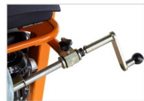
Ajuste de la profundidad de corte mediante volante
